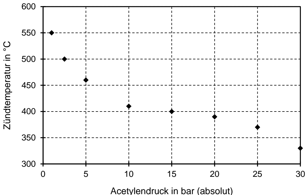
Abbildung 3: Zündtemperatur für die Auslösung einer Zerfallsreaktion von reinem Acetylen in Abhängigkeit vom Druck
